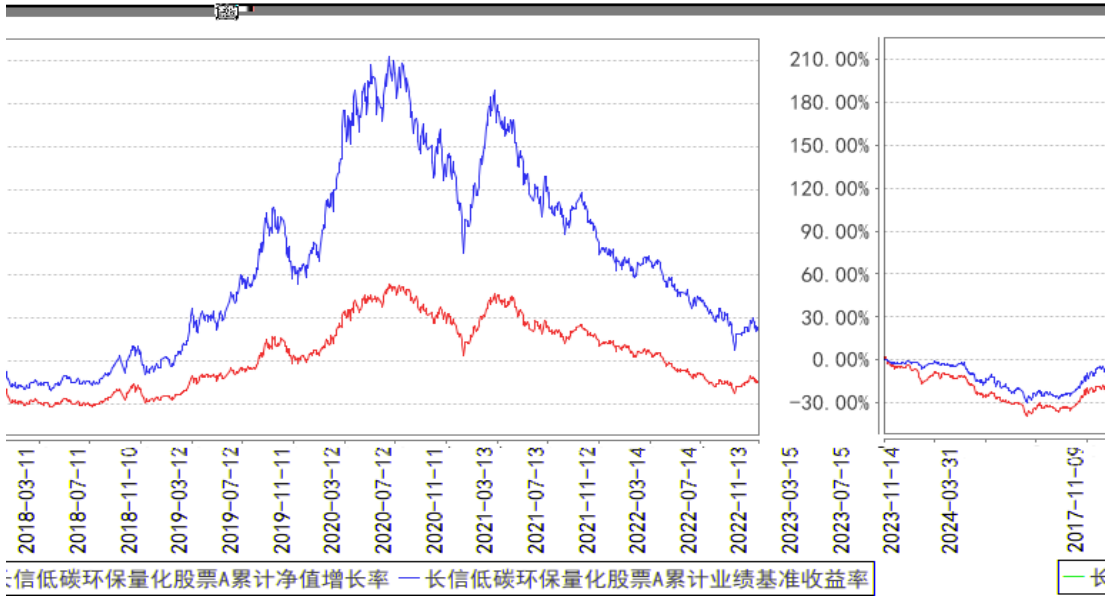
长信低碳环保量化股票A累计净值增长率与同期业绩比较基准收益率的历史走势对比
