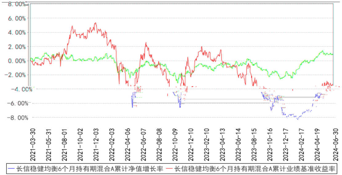
长信稳健均衡6个月持有期混合A累计净值增长率与同期业绩比较基准收益率的对比图
